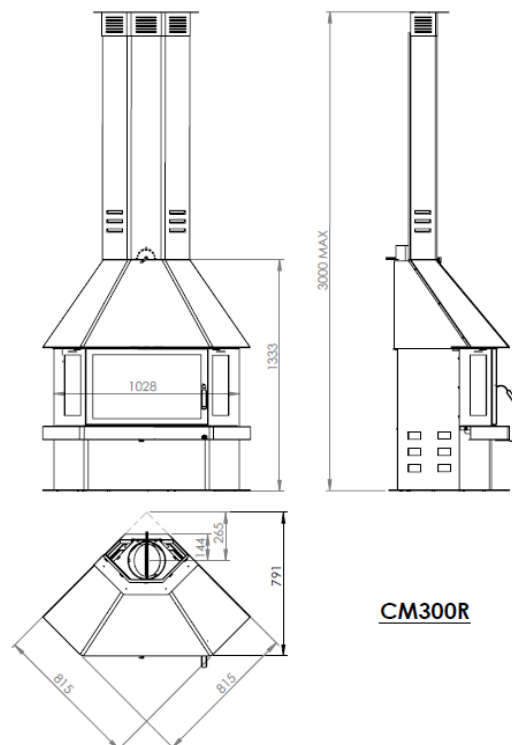
Figura n°4 - Dimensiones en mm del aparato CM-300 R
