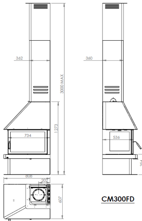
Figura n°2 - Dimensiones en mm del aparato CM-300 FD
