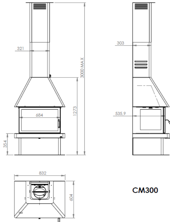
Figura n°1 - Dimensiones en mm del aparato CM-300
