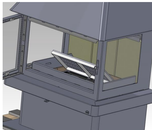
Figura nº14 - Accedemos al cenicero levantando la parrilla.
