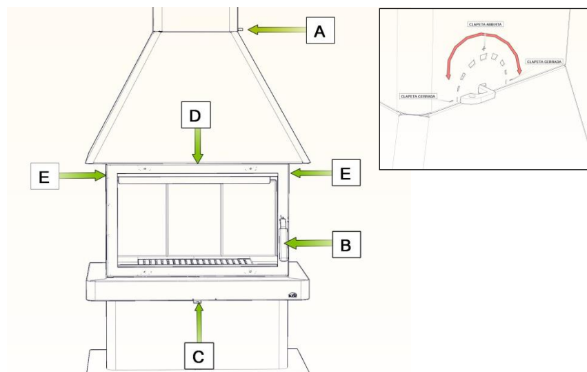
Figura n°13 - Elementos de funcionamiento del aparato
