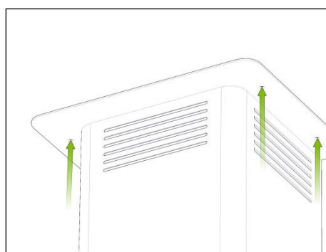
Figura nº8 - Atornillar al techo el cubre tubos superior
