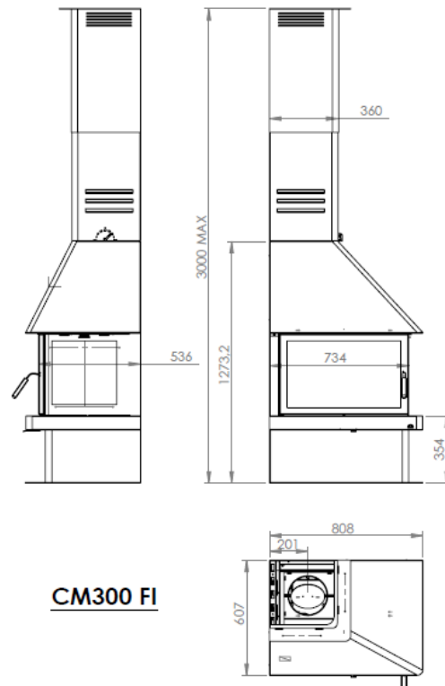
Figura n°3 - Dimensiones en mm del aparato CM-300 FI
